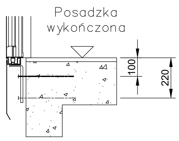
Szczegół A
